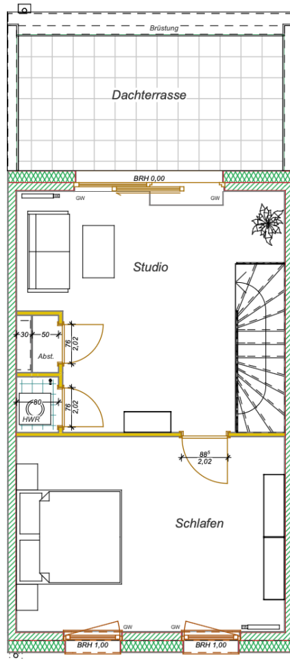
2.OG
