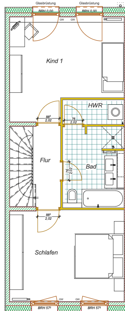
1.OG
