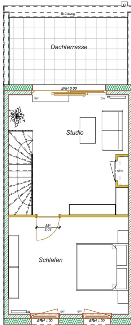
2.OG
